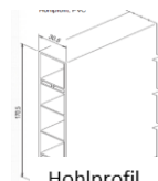
Hohlprofil 170x30 mm (8629)
