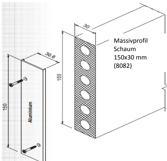
Abdeckung, Aluminium, für Profillende mit Schrauben (8201)
