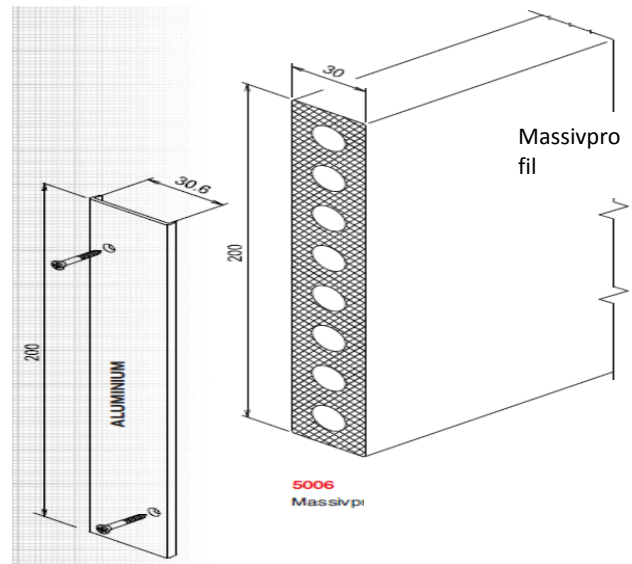
Abdeckung, Aluminium, für Profillende mit Schrauben (8200)
