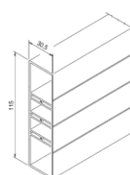
Hohlprofil 115x30 mm (8464)
