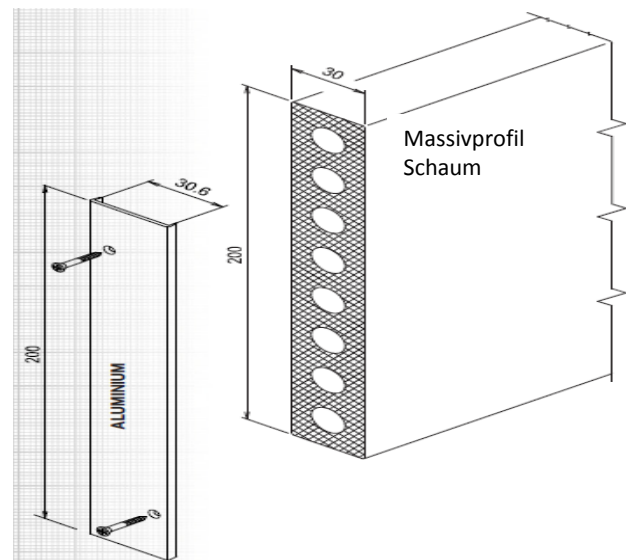
Abdeckung, Aluminium, für Profillende mit Schrauben (8200)
