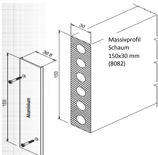
Abdeckung, Aluminium, für Profillende mit Schrauben (8201)
